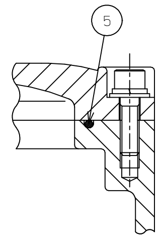
“A”部詳細図(1/2)
