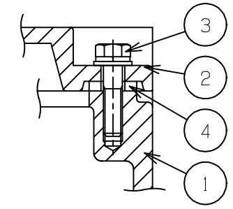
“A”部詳細図 (S=NT)
